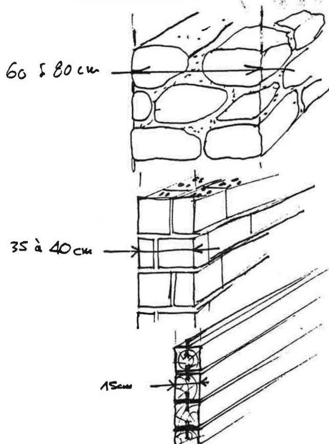
Fig. 1. - Composition d'un mur extérieur pour une inertie thermique optimale.
