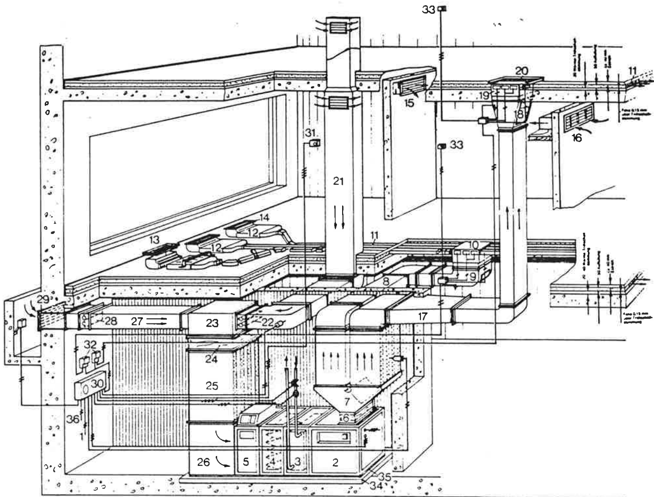
1 Wärmegerät, 2 Klima-Lüftungseinheit mit Armaturenbrett und stufenlos regelbarem Ventilator, 3 Wärmeaustauscher, 4 Feinstaubfilter, 5 Elektro-Luftfilter, 6 flexibler Flansch, 7 Zuluftverteiler mit Schöpfungen, 8 Zuluftleitung für Erdgeschoß, 9 Anschlußbogen für Revisionsöffnung, 10 Verteiler für Erdgeschoß mit Luftklappen, 11 Luftleitungen im Estrich eingegossen, 12 Zuluftauslässe mit Schalldämpfern, 13 Auflegegitter bei Teppichboden, 14 Einlegegitter bei Fliesenboden, 15 Telefoneschalldämpfer mit zwei Gittern für Umluft, 16 Kulissenschalldämpfer mit einem Gitter für Umluft bei abgehangter Decke, 17 Zuluftleitung für das Obergeschoß, 18 Übergangsstück mit Revisionsöffnung, 19 Verteiler für Obergeschoß mit Luftklappen, 20 Bodenrahmen mit Revisionsöffnung, 21 geschlossene Umluftleitung, 22 Jalousieklappe Umluft, 23 Mischkasten Umluft-Außenluft, 24 flexibler Flansch, 25 Umlufschalldämpfer, 26 Umluftanschluß, 27 Außenluftleitung, 28 Außenluftklappe dicht, 29 Außenluftgitter, 30 Regelung, 31 Wähler für Regelung, 32 Transformator für Luftklappen 220/24 Volt, 33 Raumthermostate mit Umschaltung Sommer/Winter, 34 Gerätesockel 50–60 mm hoch (bauseits), 35 Schaumgummiplatte 6 mm, 36 zum Vorlauffühler des Wärmegeräts
