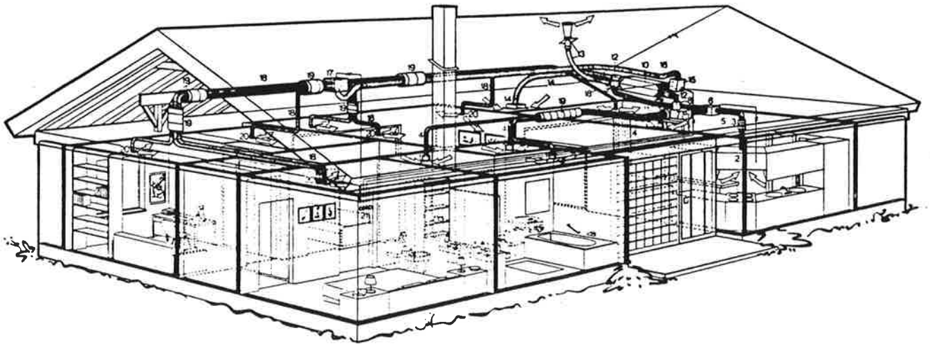
1 Abluftanschlüsse mit Filtern in den Naßräumen, 2 Küchenablufthaube mit Beleuchtung und Umschalter, 3 Deckendurchgang mit Flammenschutzkappe, 4 flexible Abluftleitungen (80 mm \phi ), 5 flexible Küchenabluftleitung (150 mm \phi ), 6 Abluftsammler mit Umschalteneinrichtung, 7 Fortluftventilator 35 W, 8 Dreiwege-Ventil für Sommerumschaltung, 9 By-pass-Leitung und T-Anschlußstück, 10 Gegenstrom-Wärmeaustauscher (Wirkungsgrad 65 %), 11 Kondenswasserabfluß, 12 Trommelluftfilter, 13 Fortluftleitung und Dachdurchführung, 14 Außenluftanschluß und Außenluftleitung 150 mm \phi , flexibel, 15 Zuluftventilator 35 W, 16 Zuluftleitung für die von der Fortluft angewärmte Außenluft (150 mm \phi ), 17 Zuluftverteiler mit Umschalteneinrichtung, 18 Zuluftleitungen, 80 mm \phi , flexibel, 19 Isolierung der Be- und Entlüftungsleitungen, 20 Zuluftdüsen, 21 Ein-Aus-Schalter für jeden Ventilator und Umschalter für Sommer- und Zeitschaltuhr
