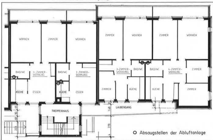
Bild 4. Für die Schweiz typischer Grundriss von Wohnungen in Mehrfamilienhaus. Abluftabsaugung in den Sanitärräumen, evtl. in der Küche; Fensterlüftung
