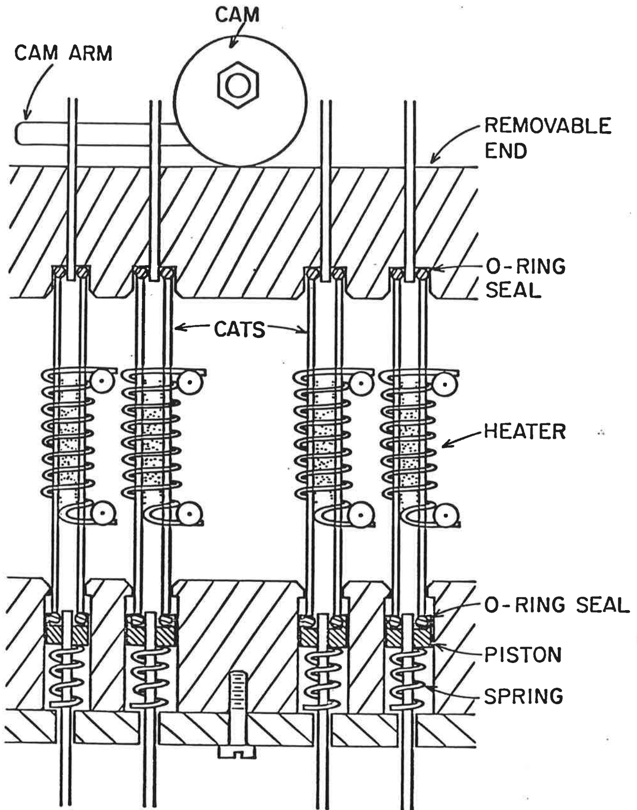
THERMAL DESORPTION APPARATUS
