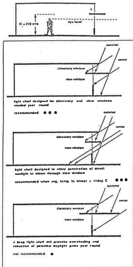
FIG. 17 Lightshelf options [18]
