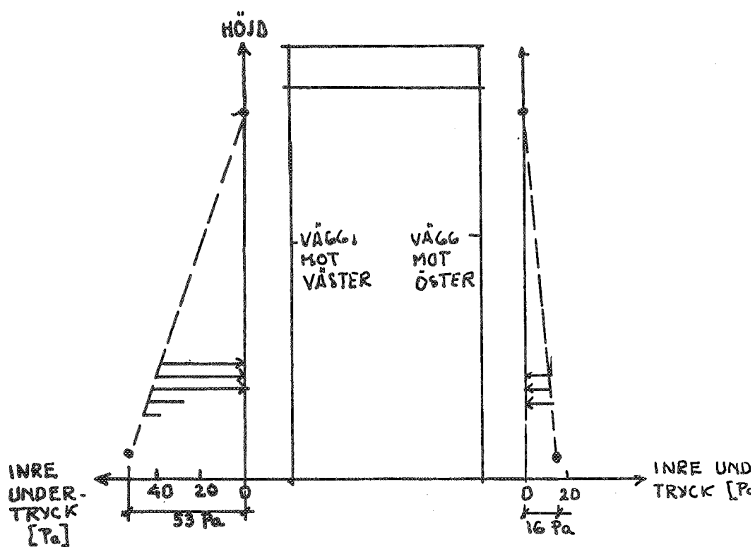
FIGUR 5.3 Uppmätta tryckskillnader över ytterväggar mot väster och öster. Tidpunkt 1977-03-10, växlande vind, temperatur +5°C.
