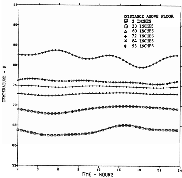
FIGURE 63e. (Bedroom 2).
